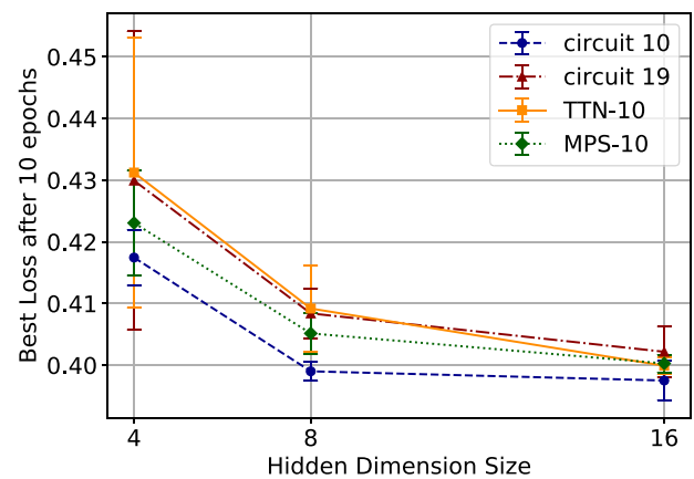
(d) Hidden dimension size ( N_D = N_Q ) comparison.
